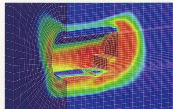
トンネル周辺の剛性低下率
